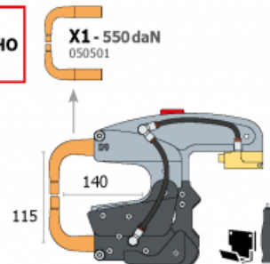
G9 + X1 - 550 daN - 022881
