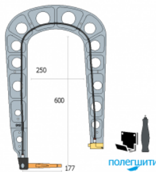
G10 - 8 bar/400 daN 067165 : 5 кг
