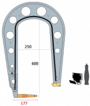
G5 - 8 bar/550 daN 022805 : 6,25 кг
