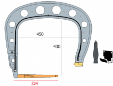
G8 - 8 bar/550 daN 022836
